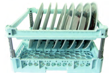
Tellerkorb für 8 große Teller mit Stoßschutz Teller max. Ø 465 mm, Grundmaß: 500 x 500 mm
